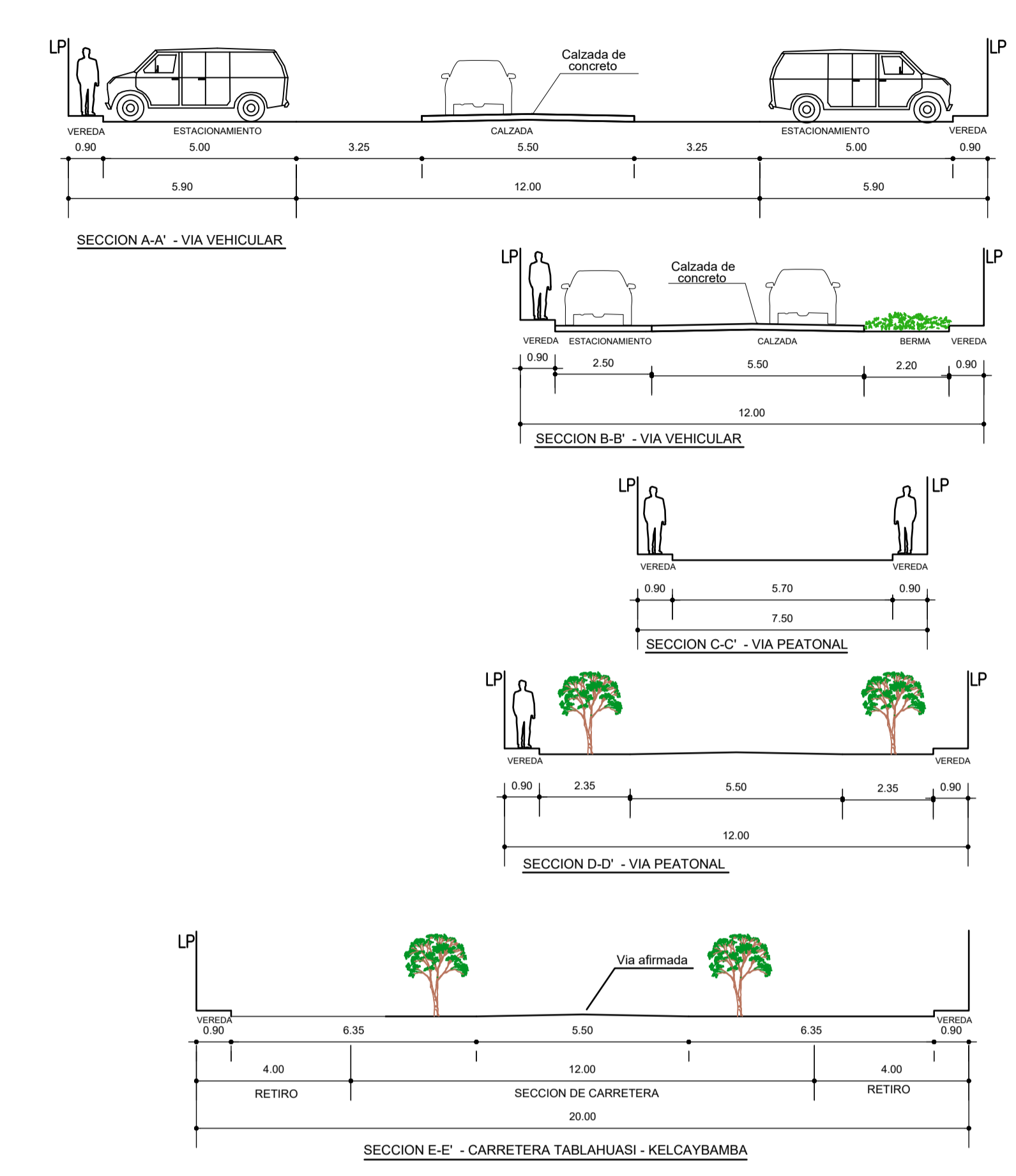
SECCION DE VIAS ESCALA : 1/125
